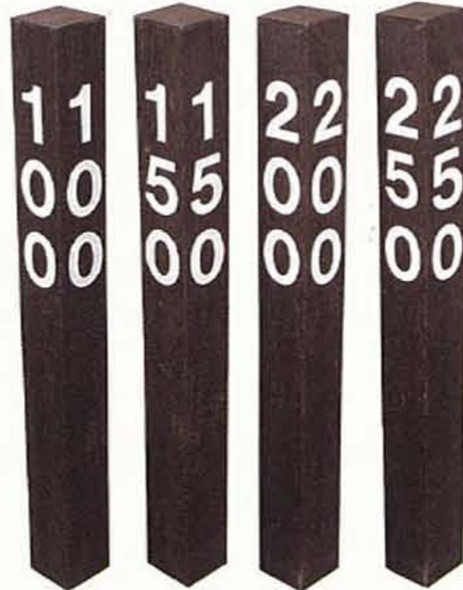
630-G 擬木角ヤード杭 擬木100×100×1000 足部スチール管48φ1500 2面彫刻
